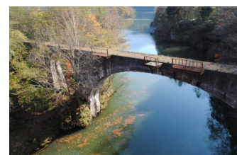
第三音更川橋りょう
